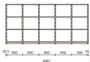
増設例 (W900mmタイプ 5連の場合)
