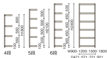
棚間隔寸法図
