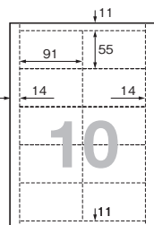
名刺(10面タイプ)寸法図
