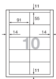
名刺(10面タイプ)寸法図
