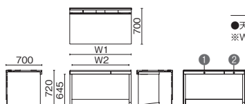
[ST-F□□□H-LP] ※図は左パネル脚/右L字脚です。
