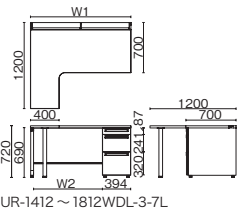
UR-1412 ~ 1812WDL-3-7L
