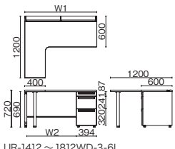
UR-1412 ~ 1812WD-3-6L
