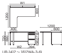
UR-1412 ~ 1812WA-3-6L
