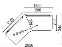
スタート用 XL-135S
