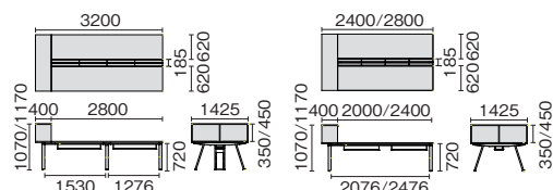
GE-N2414KS4 T2 / SBK 収納内向き装着時
