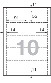
名刺(10面タイプ)寸法図
