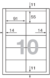
名刺(10面タイプ)寸法図
