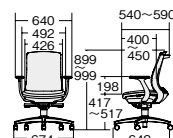
ローバック固定肘
