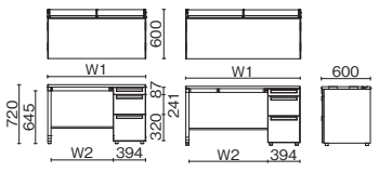
US-107 ~ 127D-3 US-147 ~ 167D-3 US-107 ~ 127DL-3 US-147 ~ 167DL-3 ※標準収納タイプは①、多量収納タイプは②
