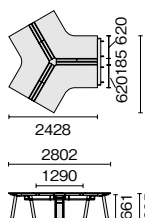
GE-N1214WJ-12 WM/W4
