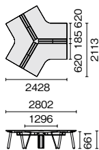
GE-N1214WB-12 WM/W4
