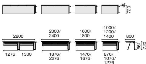
GE-N□□8KJ
