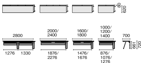
GE-N□□7KJ
