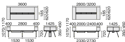
GE-N2414WS4 T2 / BK 収納内向き装着時
