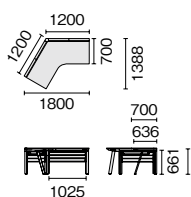
GE-N127K-12 WM/W4
