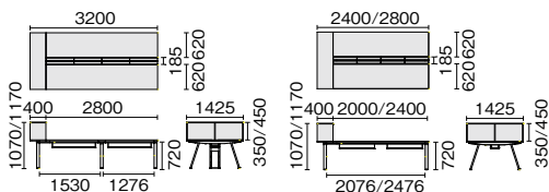
GE-N2414KS4 T2 / BK 収納内向き装着時
