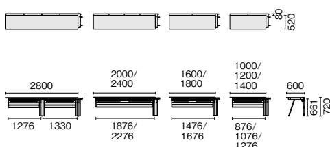
GE-N□□6KJ
