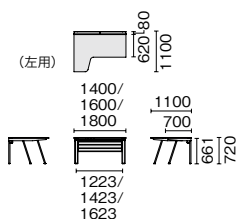
GE-N167RL WM/W4 (左用)
