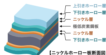
【ニッケルホーロー板断面図】
